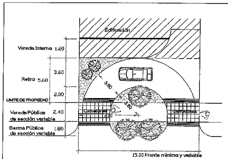
PLANO DE LA BAHIA 6 REFUGIO VEHICULAR
